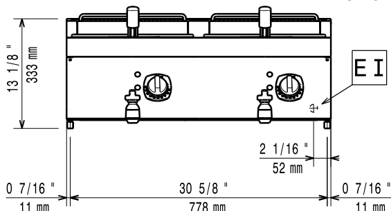
Előlnézet
