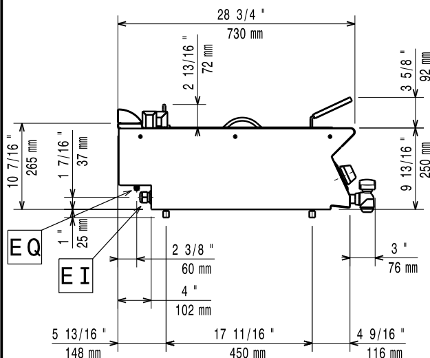
Oldalnézet
